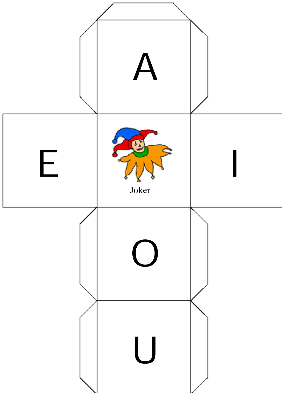
Vokal – Würfel
